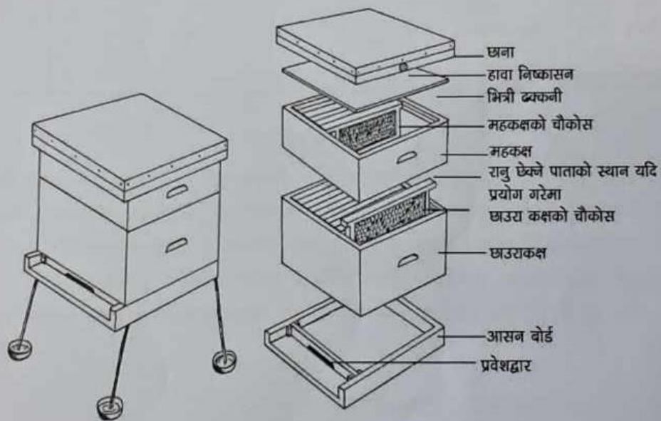
चित्र: न्युटन वी टाइप घर (साइज तथा आकार र स्पेसिफिकेशन न्युटन वी टाइप घरको संलग्न/तोकिएको प्रचलित नर्मस अनुसार हुनुपर्ने)
